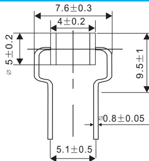
Dimensions(mm)尺寸
